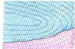
Fig. 5. Überspringen der Schieferung des Gneisses auf den C-förmig gebogenen Kalk am oberen Kalkkeil d. Jungfrau
